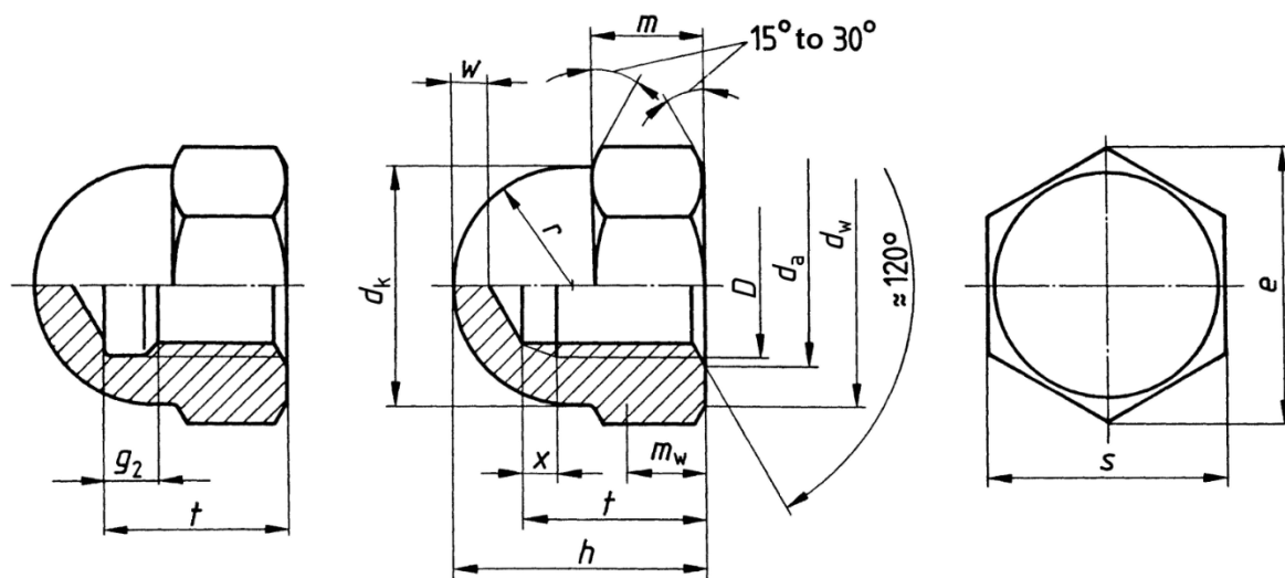
DIN 1587 Hexagon Domed Cap Nut (Dome Nut)
